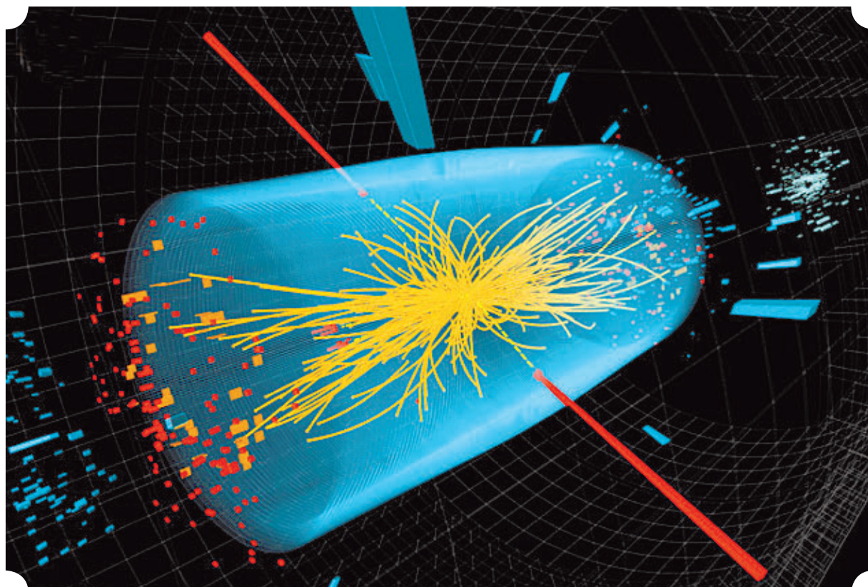
Imagen donde se representa la aparición del Bosón de Higgs después de una colisión de protones, detectada por el experimento Atlas del LHC.
