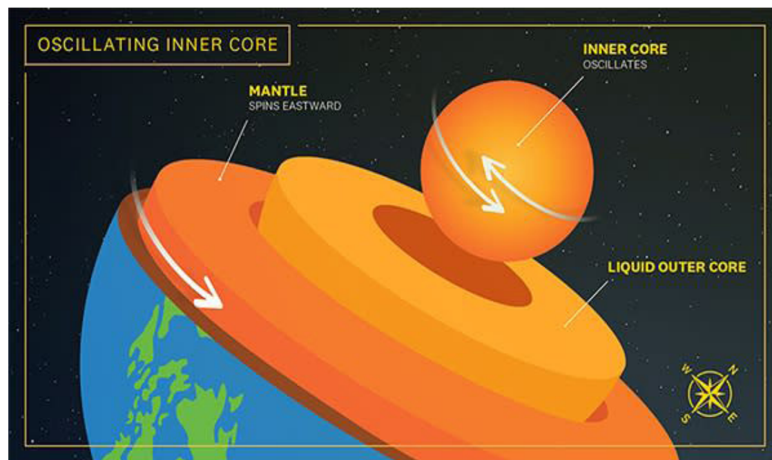
Un diagrama de cómo el núcleo de la Tierra oscila.
