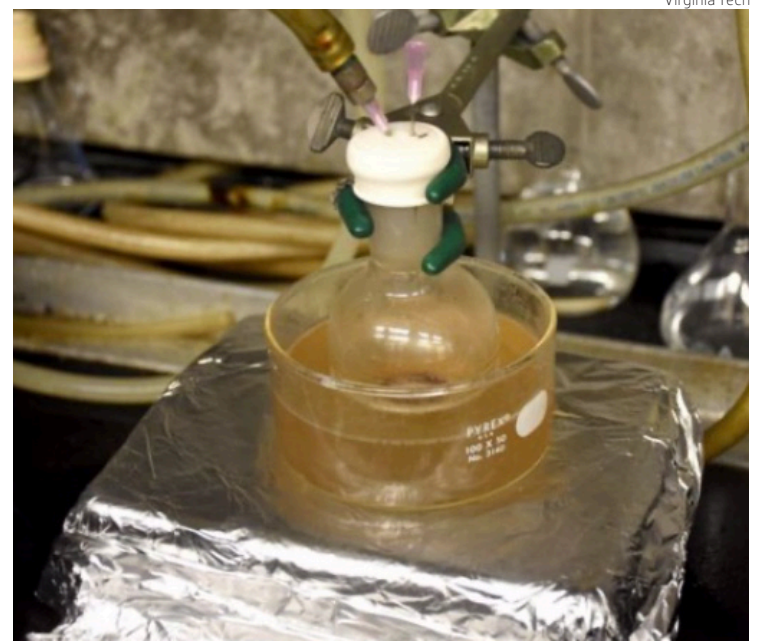
Matraz lleno de ceras generadas a partir de residuos de polipropileno.
