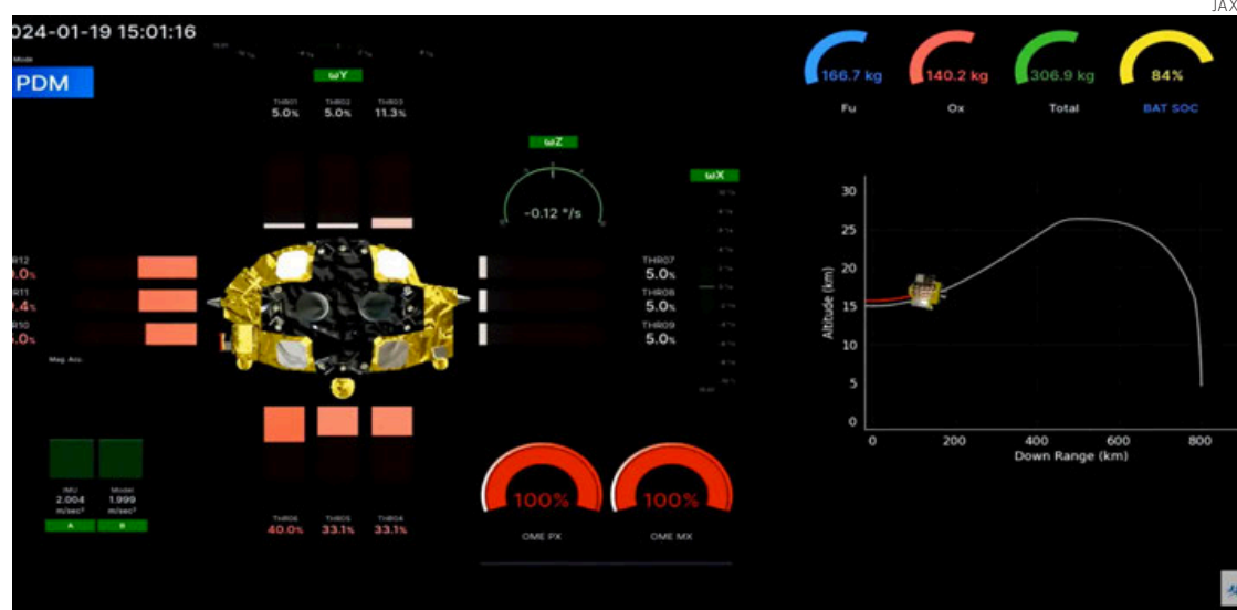
La telemetría que confirmó el aterrizaje del módulo japonés SLIM en la Luna.
